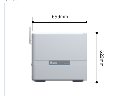
寸法図
