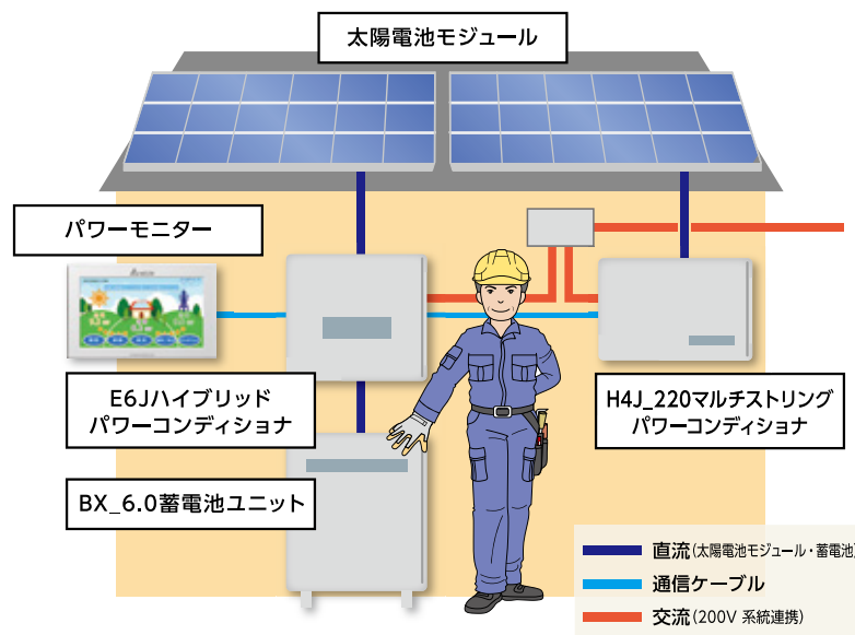
9.9kW システム構成例
