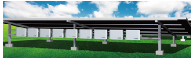
「H5.5J_223」を9台、傾斜角10度、6インチセル60直モジュール横置き4段架台(積雪50cm)に配置したイメージ図
